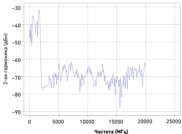
Гармоники при уровне +20 дБм, опция 520 (изм.)
