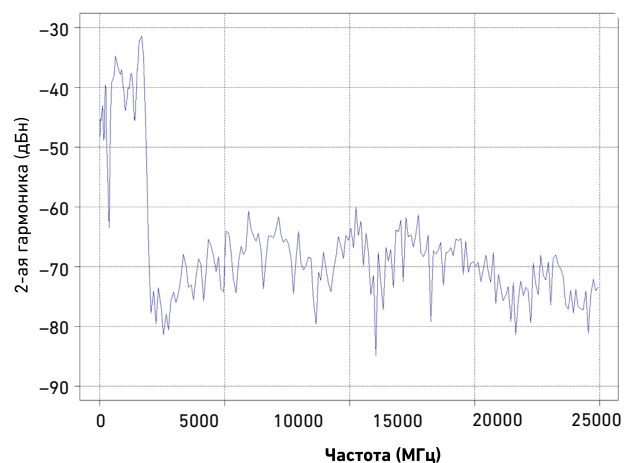
Гармоники при уровне +20 дБм, опция 540 (изм.)
