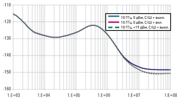
Зависимость L(f) [дБн/Гц] от отстройки от частоты несущей
