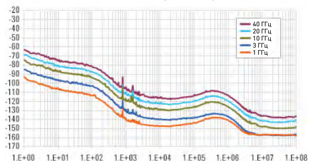
Зависимость L(f) [дБн/Гц] от отстройки от частоты несущей
