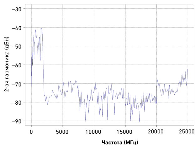
Гармоники при уровне +10 дБм, опция 540 (изм.)
