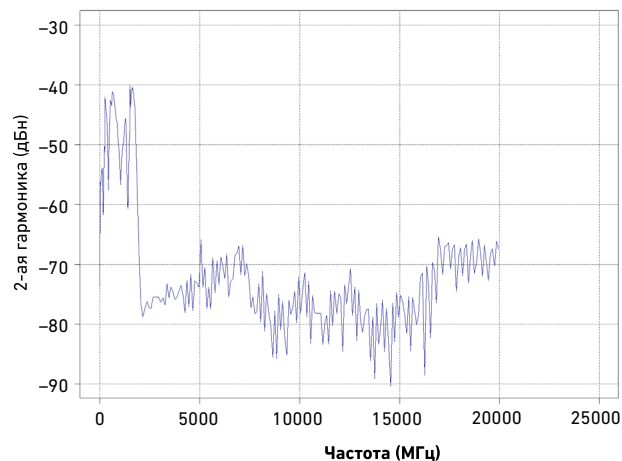
Гармоники при уровне +10 дБм, опция 520 (изм.)
